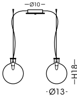
793.2L Sospensione / Hanging lamp vetro/glass Ø13 cm - cavo/cable 250 cm
