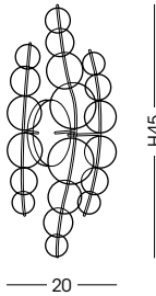
.2L Applique / Wall lamp L20 cm - P16 cm - H45 cm 2 G9 x max 42W 230V CE IP20 1m
