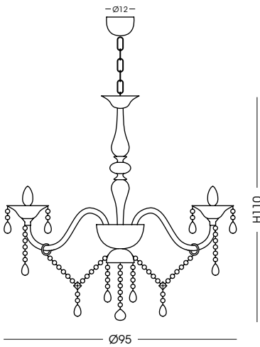
684.12L Lampadario / Chandelier Ø95cm - H110 cm - catena/chain 50 cm 12 E14 x max 40W 220-240V CE IP20 1m
