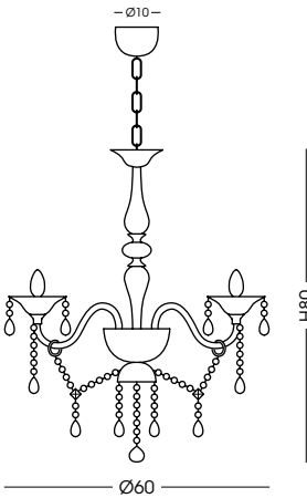
684.3L Lampadario / Chandelier Ø60 cm - H80 cm - catena/chain 50 cm 3 E14 x max 40W 220-240V CE IP20 1m
