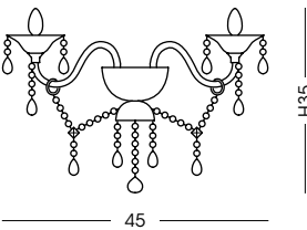
AP681.2L Applique / Wall lamp L45 cm - P25 cm - H35 cm 2 E14 x max 40W 220-240V CE IP20 1m
