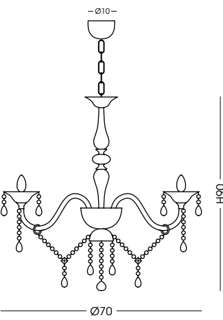
684.6L Lampadario / Chandelier Ø70 cm - H90 cm - catena/chain 50 cm 6 E14 x max 40W 220-240V CE IP20 1m
