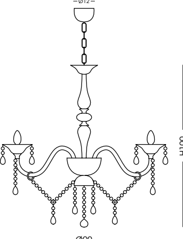
684.8L Lampadario / Chandelier Ø90cm - H100 cm - catena/chain 50 cm 8 E14 x max 40W 220-240V CE IP20 1m
