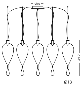
803.5L Sospensione / Hanging lamp vetro/glass Ø13 cm - cavo/cable 250 cm 5 G9 x max 42W 230V CE IP20 1m
