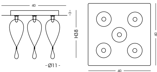
809.5L Plafoniera / Ceiling lamp vetro/glass Ø11 cm - H 38 cm 5 G9 x max 42W 230V CE IP20 1m
