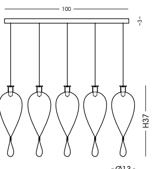
807.5L Binario a soffitto / Ceiling track vetro/glass Ø13 cm - cavo/cable 150 cm 5 G9 x max 42W 230V CE IP20 1m
