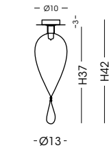
806.1L Plafoniera / Ceiling lamp vetro/glass Ø13 cm - H 42 cm 1 G9 x max 42W 230V CE IP20 1m
