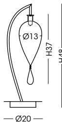
LU804.1L Lumetta/ Table lamp vetro/glass Ø13 cm - H 48 cm 1 G9 x max 42W 230V CE IP20 1m
