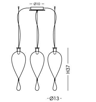
803.3L Sospensione / Hanging lamp vetro/glass Ø13 cm - cavo/cable 250 cm 3 G9 x max 42W 230V CE IP20 1m
