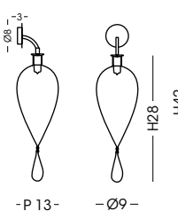
AP801.1L Applique / Wall lamp vetro/glass Ø9 cm - H 42 cm 1 G9 x max 42W 230V CE IP20 1m
