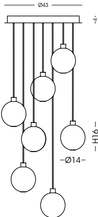
1299.7L Plafoniera / Ceiling lamp vetro/glass Ø14 cm - cavo/cable 150 cm 7 G9 x max 33W 230V CE IP20 1m
