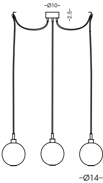
1293.3L Sospensione / Hanging lamp vetro/glass Ø14 cm - cavo/cable 250 cm 3 G9 x max 33W 230V CE IP20 1m
