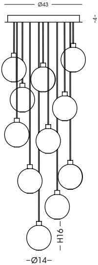
1299.11L Plafoniera / Ceiling lamp vetro/glass Ø14 cm - cavo/cable 150 cm 11 G9 x max 33W 230V CE IP20 1m
