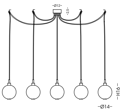
1293.5L Sospensione / Hanging lamp vetro/glass Ø14 cm - cavo/cable 250 cm 5 G9 x max 33W 230V CE IP20 1m
