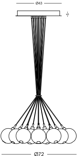
1292.19L Plafoniera / Ceiling lamp vetro/glass Ø14 cm - Cavo/Cable 250 cm 19 G9 x max 33W 230V CE IP20 1m
