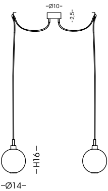
1293.2L Sospensione / Hanging lamp vetro/glass Ø14 cm - cavo/cable 250 cm 2 G9 x max 33W 230V CE IP20 1m
