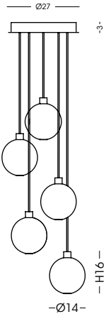
1299.5L Plafoniera / Ceiling lamp vetro/glass Ø14 cm - cavo/cable 150 cm 5 G9 x max 33W 230V CE IP20 1m
