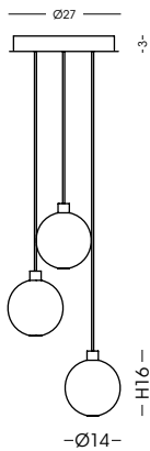
1299.3L Plafoniera / Ceiling lamp vetro/glass Ø14 cm - cavo/cable 150 cm 3 G9 x max 33W 230V CE IP20 1m
