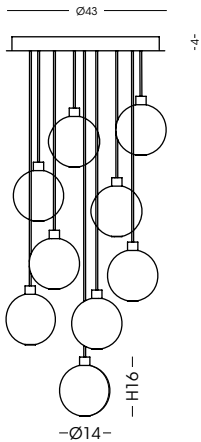
1299.9L Plafoniera / Ceiling lamp vetro/glass Ø14 cm - cavo/cable 150 cm 9 G9 x max 33W 230V CE IP20 1m
