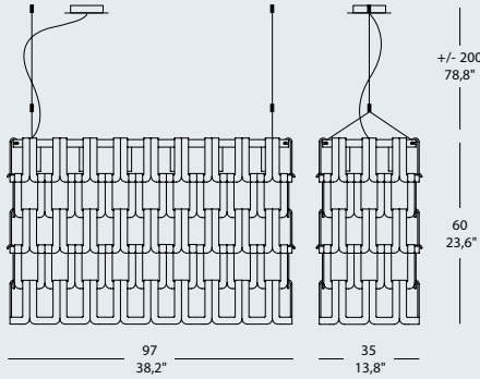
TESSUTI SO 90 MAXI 12 x MAX 42W G9 alo. ENERGY SAVER IP 20
