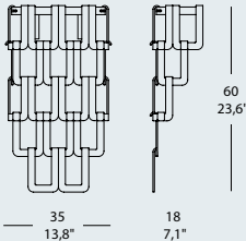
TESSUTI PA 30 MAXI 2 x MAX 42W G9 alo. ENERGY SAVER IP 20
