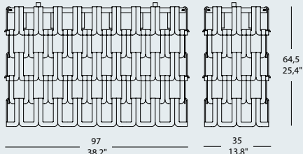
TESSUTI PL 90 MAXI 12 x MAX 42W G9 alo. ENERGY SAVER IP 20
