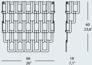
TESSUTI PA 60 MAXI 4 x MAX 42W G9 alo. ENERGY SAVER IP 20
