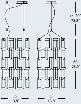
TESSUTI SO 30 MAXI 4 x MAX 42W G9 alo. ENERGY SAVER IP 20
