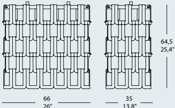
TESSUTI PL 60 MAXI 8 x MAX 42W G9 alo. ENERGY SAVER IP 20
