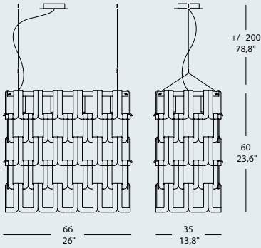
TESSUTI SO 60 MAXI 8 x MAX 42W G9 alo. ENERGY SAVER IP 20
