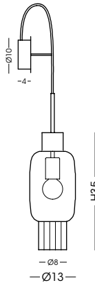
AP1361.1L Applique / Wall lamp vetro/glass Ø13 cm - cavo/cable 50 cm 1 E27 x max 42W 220-240V CE IP20 1m
