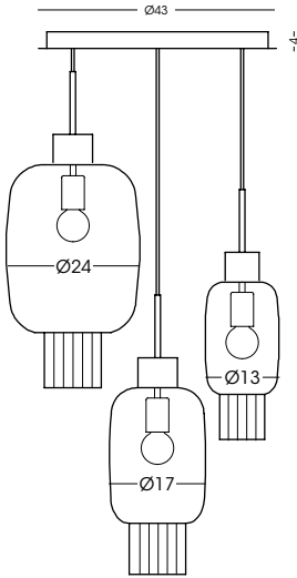
1369MX.3L Plafoniera / Ceiling lamp vetro/glass Ø13/17/24 cm - cavo/cable 150 cm 1 E27 x max 42W 2 E27 x max 70W 220-240V CE IP20 1m
