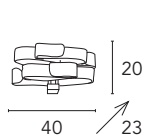
Gloria 1360/A2L 2 x max 60W E14 230V CE V □
