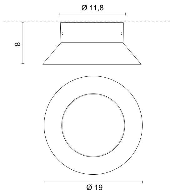
Dimensioni - Dimensions
