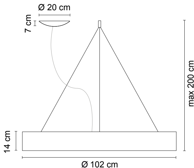
Dimensioni - dimensions
