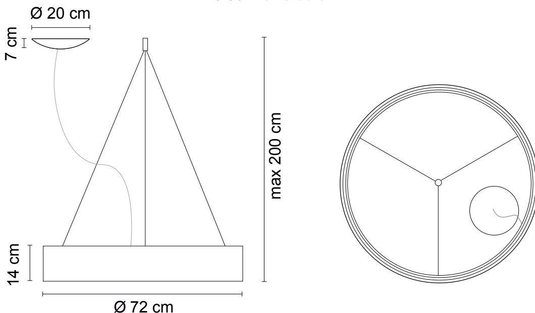
Dimensioni - dimensions
