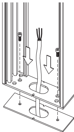
auf Erdspeiß oder Erdanker on ground spike or ground anchor
