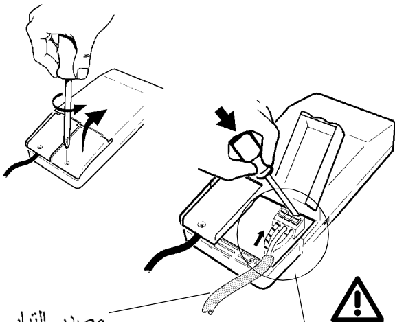
مصدر التيار ALIMENTAZIONE POWER SUPPLY CEBADOR
