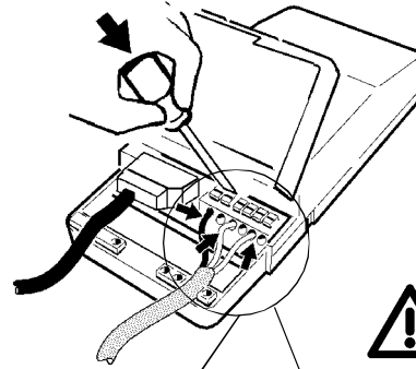
مصدر التيار ALIMENTAZIONE POWER SUPPLY CEBADOR
