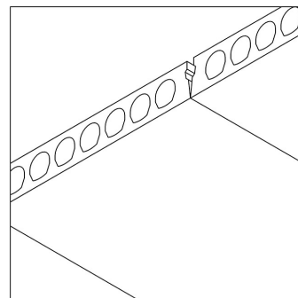
Многослойная железобетонная плита
