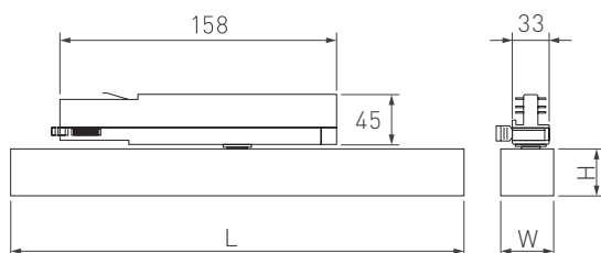
Рис. 1. Чертеж и габаритные размеры
