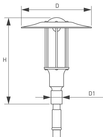
Рис. 1. Чертеж и габаритные размеры
