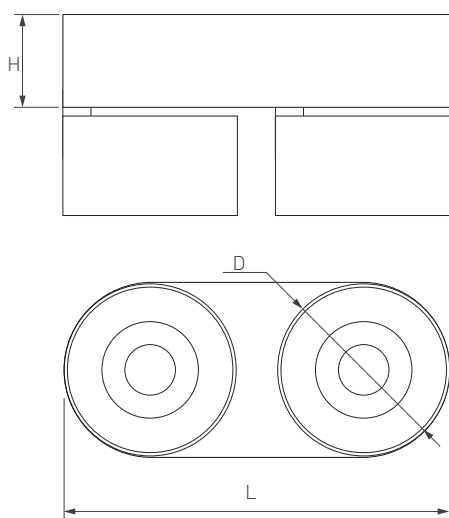
Рис. 1. Чертеж и габаритные размеры
