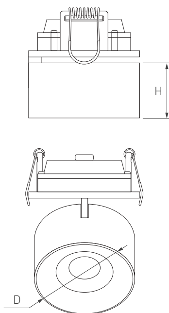
Рис. 1. Чертеж и габаритные размеры
