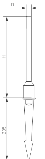
Рис. 1. Чертеж и габаритные размеры
