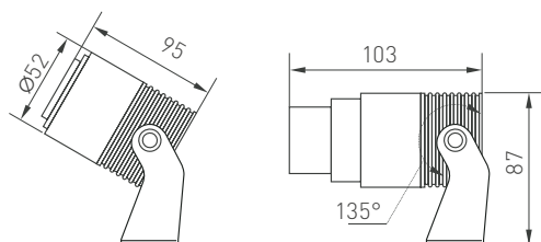
Рис. 1. Чертеж и габаритные размеры
