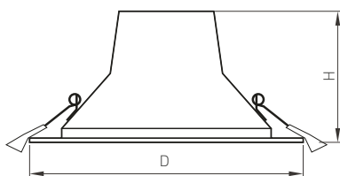
Рис. 1. Чертеж и габаритные размеры
