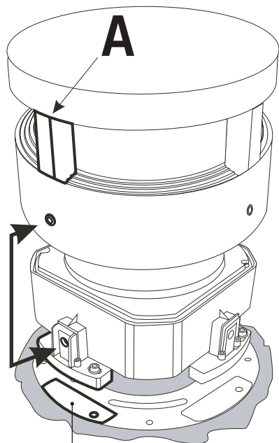
S.5203 FLANGIA / FLANGE
