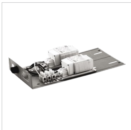
Монтажная плата
